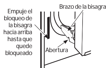
Empuje el bloqueo de la bisagra hacia arriba hasta que quede bloqueado Abertura Brazo de la bisagra Apoye la abertura en el extremo inferior de la ranura de la bisagra
